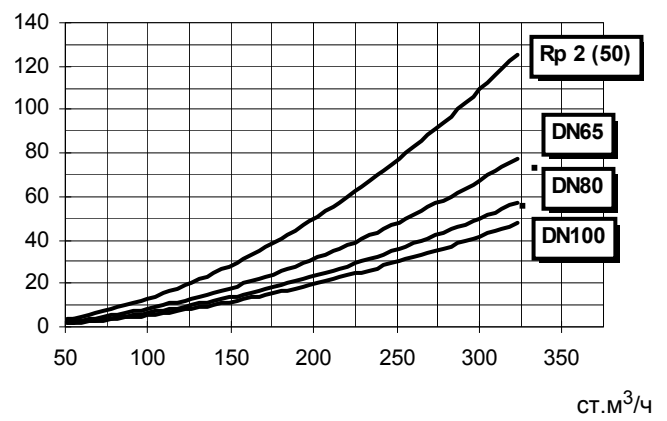
HR512A
