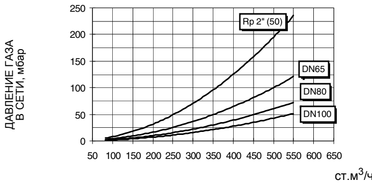
HR525A Rp2
