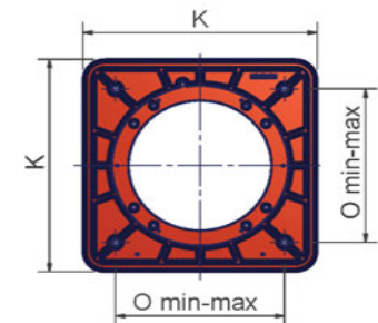
Фланец горелки
